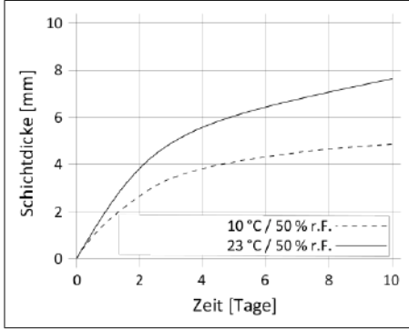
Diagramm 1: Durchhärtengeschwindigkeit Sikaflex®-521 FC
